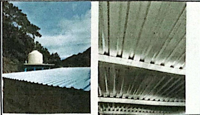
Foto 1: sustitución de lámina troquelada aluzinc calibre 28 y sustitución de estructura de soporte de metal en cocina escolar
